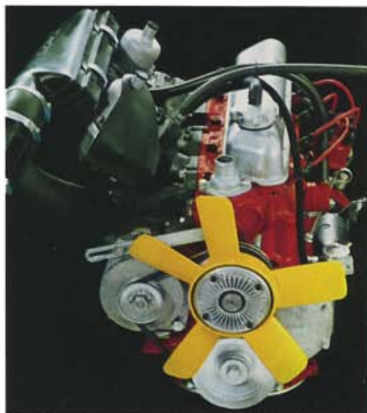
B 20 B. 2 liters, 4-cylindrig, 118 hk SAE. Avgasrening som standard. (Bilden visar motorn i utförande för Volvo 140-serien.)
